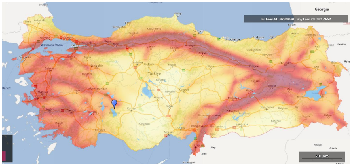
Şekil 2-7 Alt Proje Alanı Sınırları İçerisinde Yer Alan Aktif Fay Hatları
