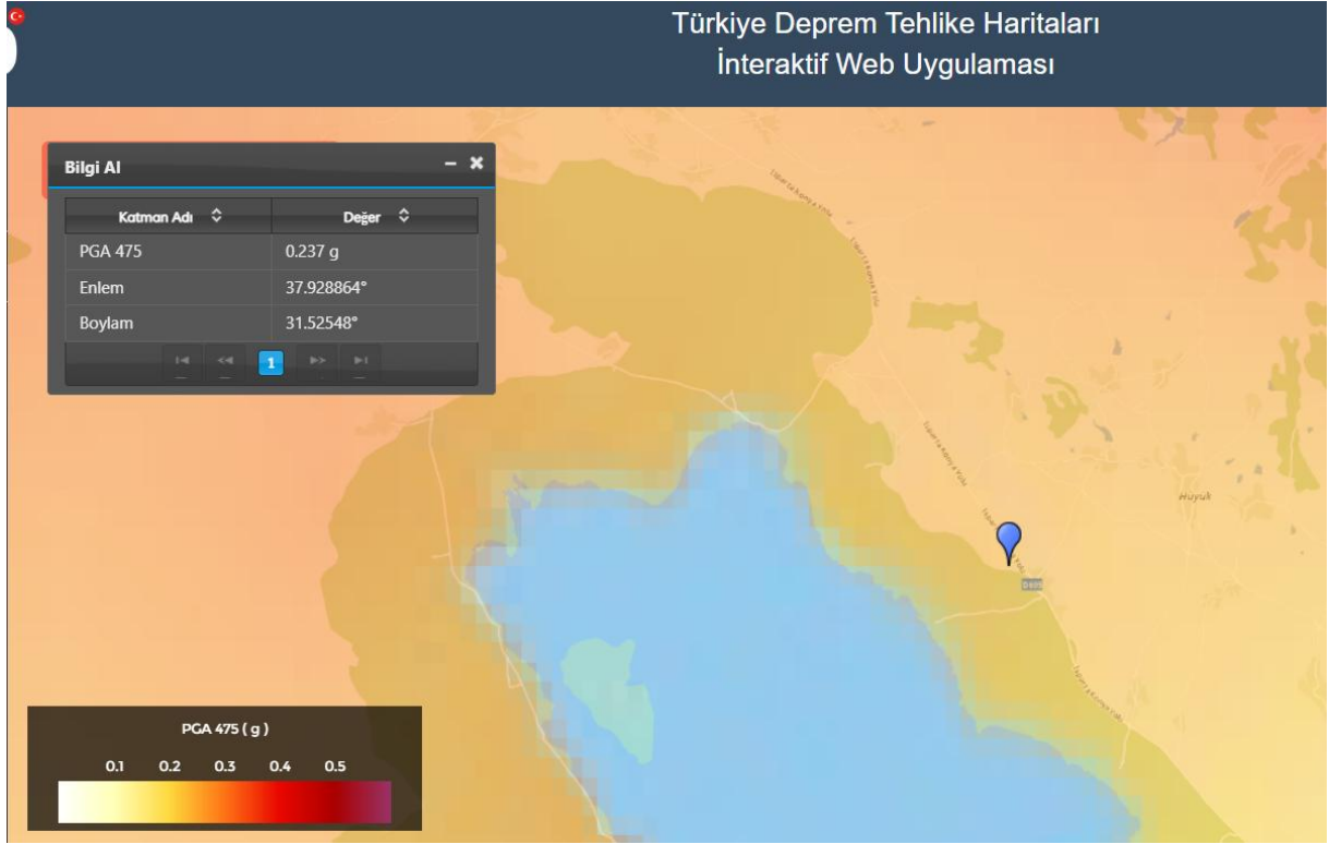
Şekil 2-6 Alt Proje Alanının Deprem Risk Haritası
