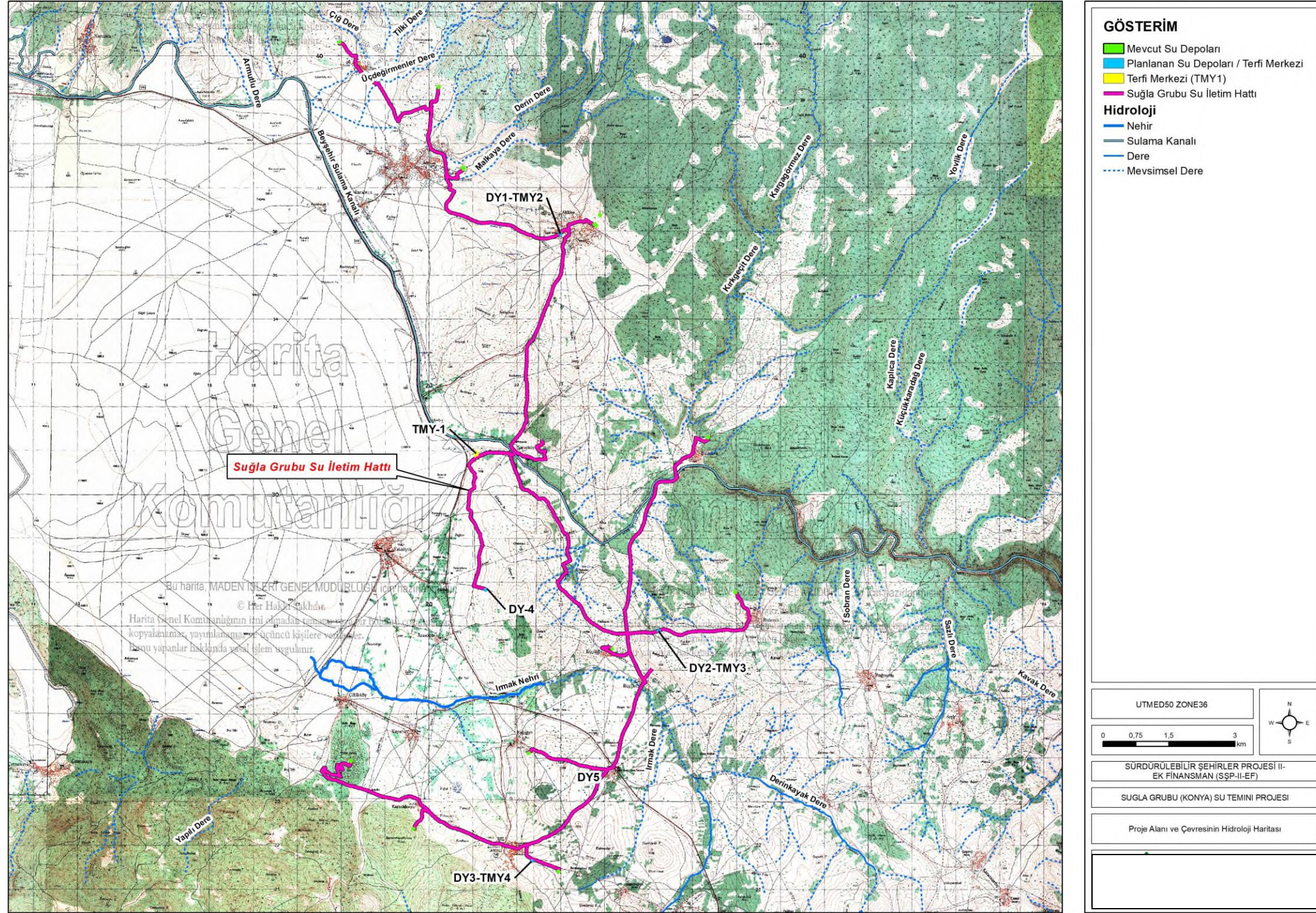
Şekil 4-8 Projenin Hidrojeoloji Haritası
