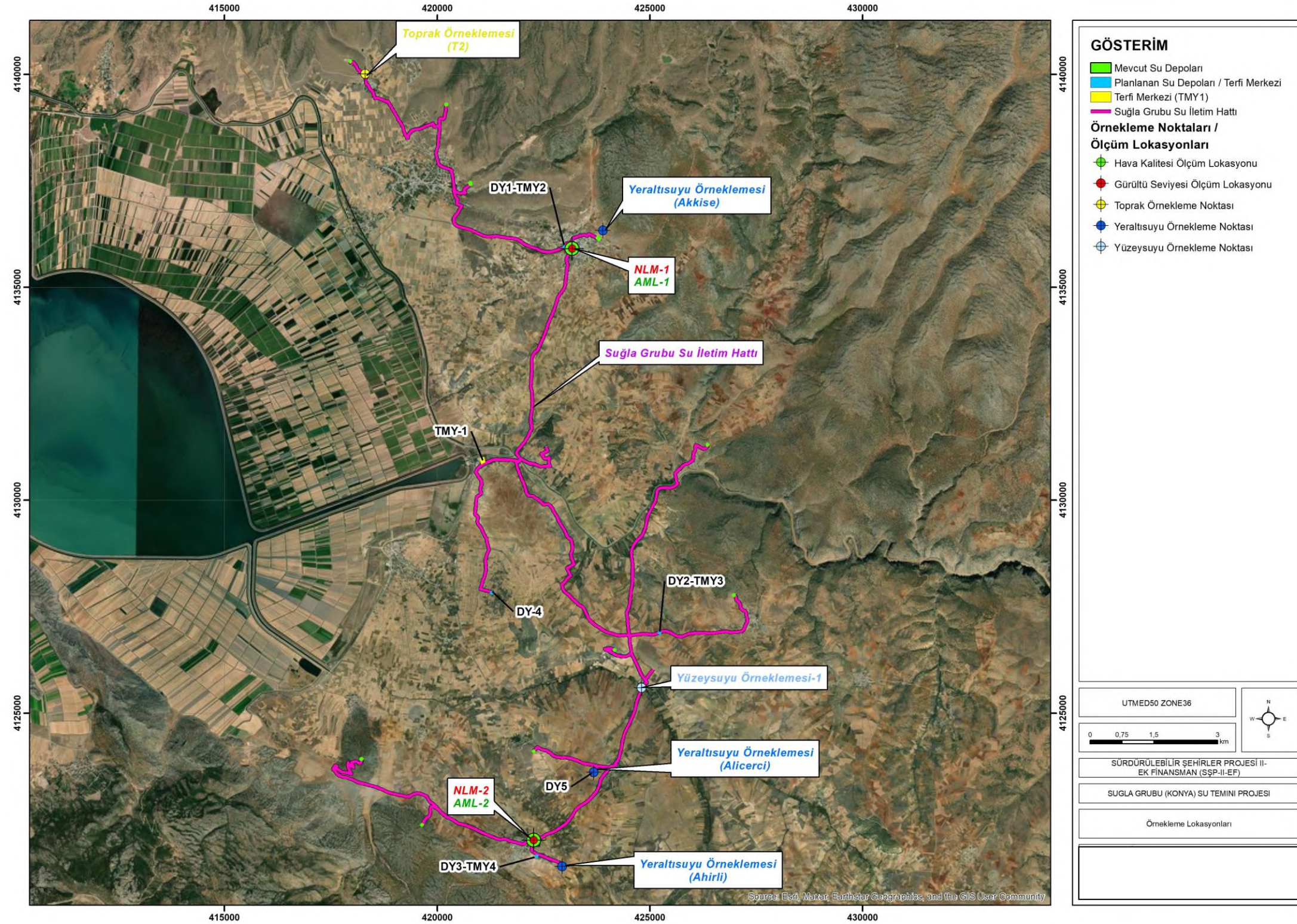
Şekil 4-10. Örneklemeler Konumları
