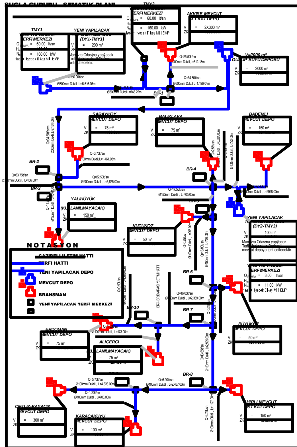
Şekil 3-3.Projenin Şematik Planı
