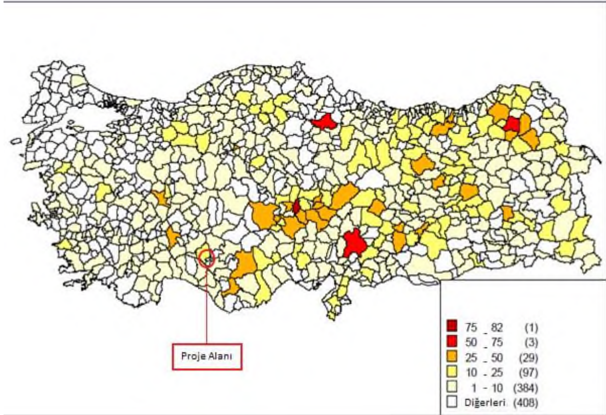
Şekil 4-3 Ahırılı ve Yalılıyük İlçelerinin Kaya Düşmesi Haritası
