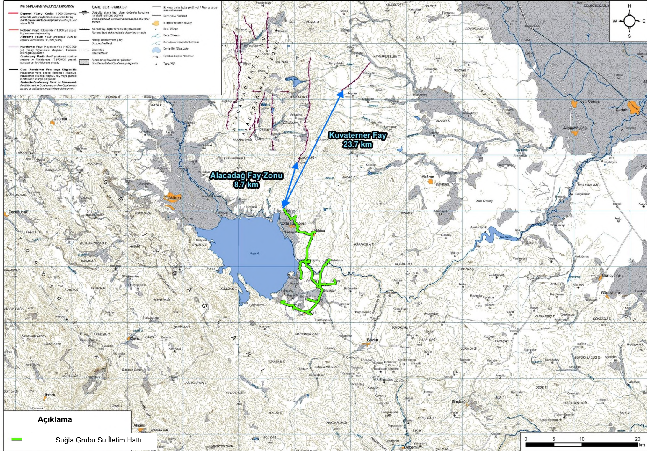
Şekil 4-6 Projenin Aktif Fay Hattı Haritası
